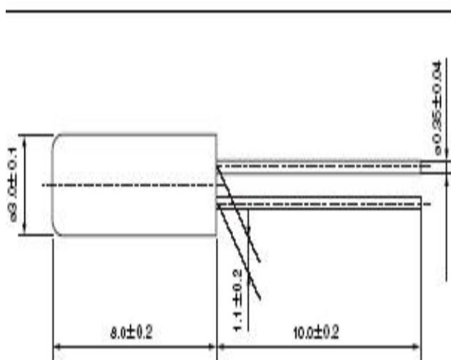
OUTLINE DIMENSIONS(UNIT:mm) 外形尺寸 (单位: mm)
