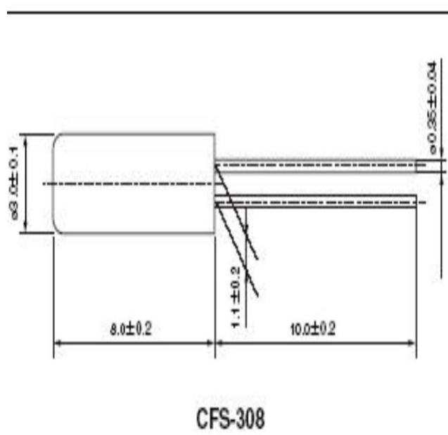
OUTLINE DIMENSIONS(UNIT:mm) 外形尺寸 (单位: mm)
