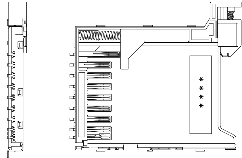
コネクタ上面(板金外し状態)
