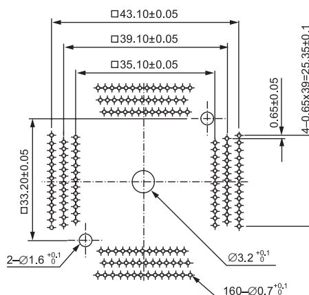
QFP IC201-1604-006 (160 Pins)
