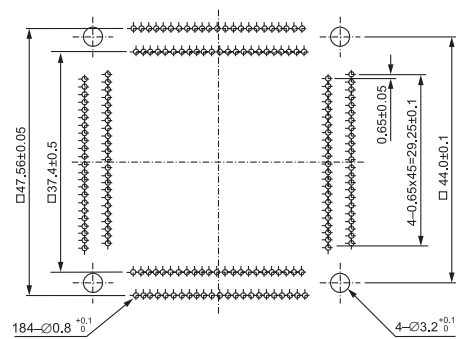
IC51-1844-1148-1 (184 Pins)
