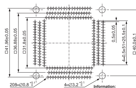
IC51-2084-1052-* 2) (208 Pins)
