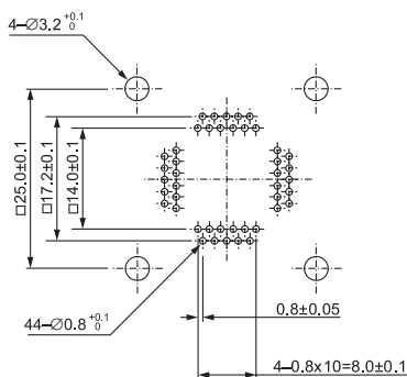
IC51-467-KS11787 (44 Pins)
