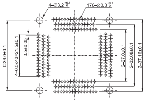
IC51-1764-1505 (176 Pins)
