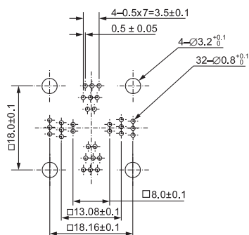
IC51-0324-805 (32 Pins)
