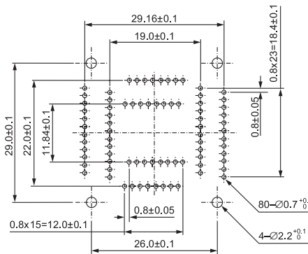
IC51-819-KS12720 (80 Pins)
