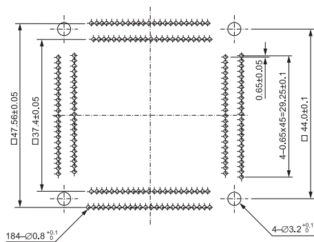
IC51-1844-1541 (184 Pins)
