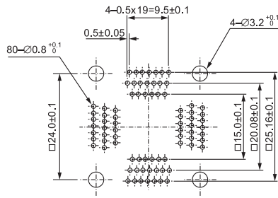
IC51-0804-711 (80 Pins)
