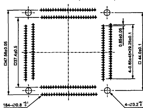
IC51-1844-1148-1 (184 Pins)
