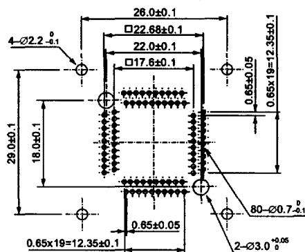
IC51-0804-956-2 (80 Pins)
