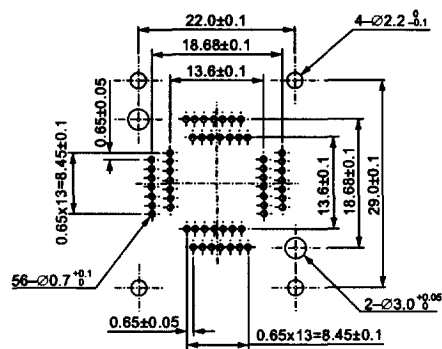
IC51-0564-680 (56 Pins)
