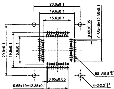
IC51-0804-956-2 (80 Pins)
