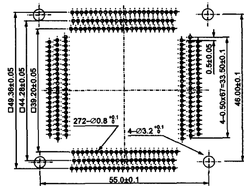
IC51-3044-1471-2 (304 Pins)
