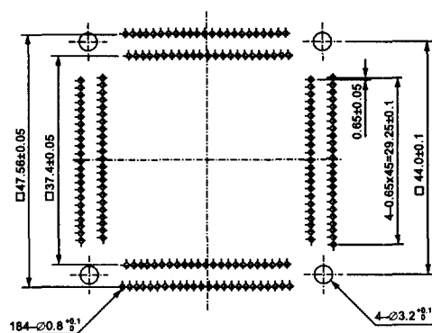
IC51-1844-1541 (184 Pins)
