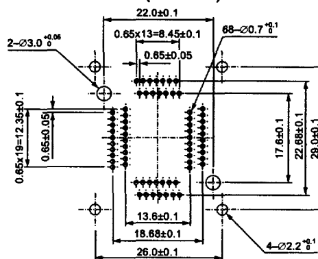
IC51-0684-734 (68 Pins)
