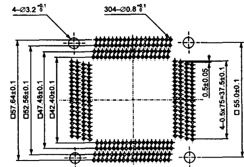
IC51-3044-1471-5 (304 Pins)
