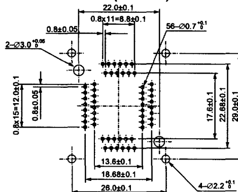
IC51-0564-924 (56 Pins)
