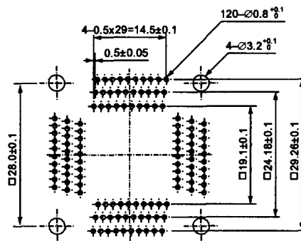
IC51-1204-1652 (120 Pins)
