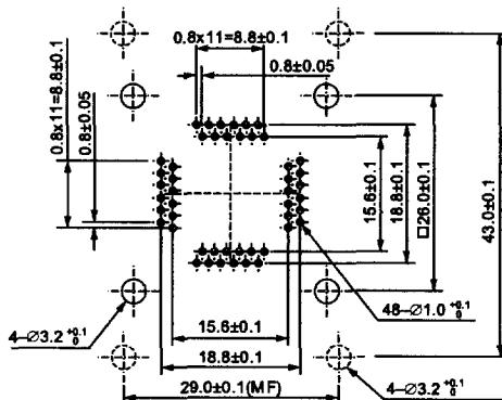
IC51-0484-081 (48 Pins)
