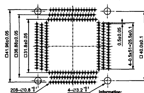
IC51-2084-1052-* 2) (208 Pins)
