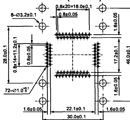
IC51-0724-698 (72 Pins)
