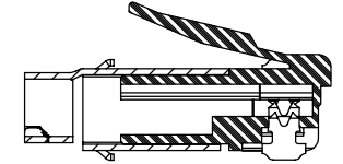
SCHNITT C-C MAßSTAB 3 : 1
