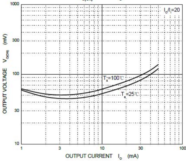
V_{OL(on)} — I_o
