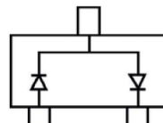
BAS40-04
