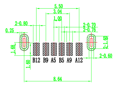
PCB板参考图
