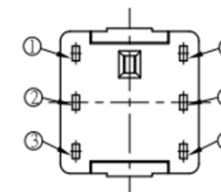
A-A VIEW
