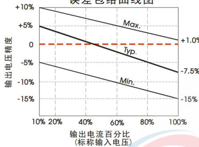
3.3VDC 输出 误差包络曲线图
