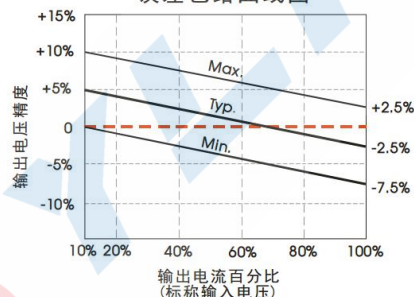
其他输出 误差包络曲线图
