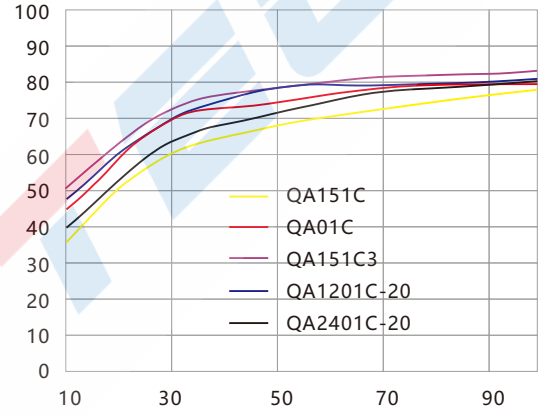
效率Vs输出负载 (标称电压输入)
