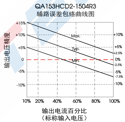
图 7 (辅路误差包络曲线)
