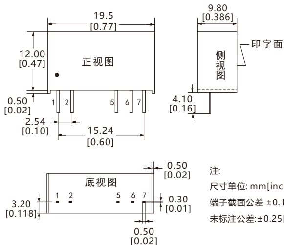
外观尺寸
