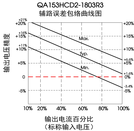
图 11 (辅路误差包络曲线)
