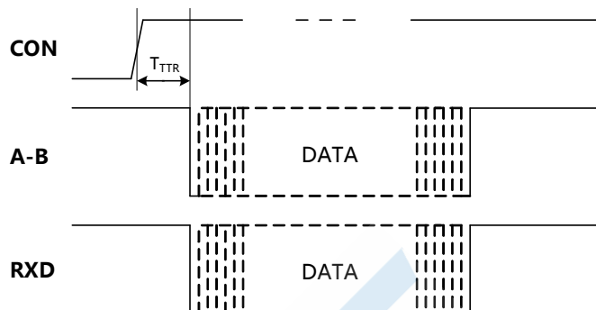
图 2. RSM(3)485PCHT模块数据接收时序图
