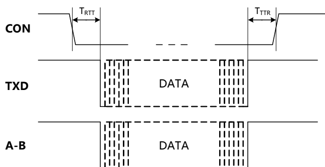
图 1. RSM(3)485PCHT模块数据发送时序图
