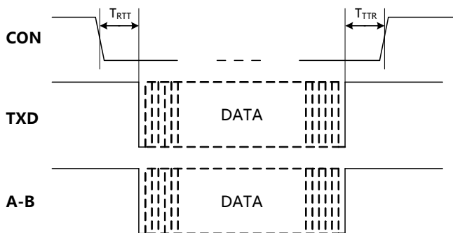
图 1. RSM(3)485PCT模块数据发送时序图
