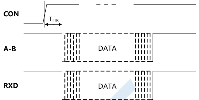
图 2. RSM(3)485PCHT模块数据接收时序图
