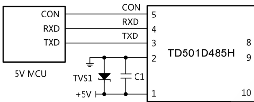
图 3.MCU 5V供电应用电路
