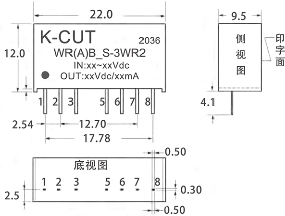
1) 外观尺寸 (单位: mm,公差: xx \pm 0.25 )
