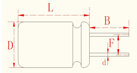
引线切脚成型 B 图
