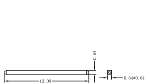
PIN针规格
