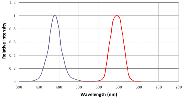
光谱分布特性曲线 Spectrum Distribution (Ta=25°C)
