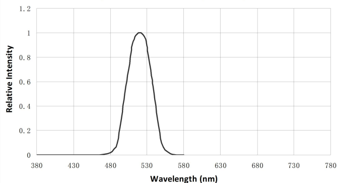
光谱分布特性曲线 Spectrum Distribution (Ta=25°C)
