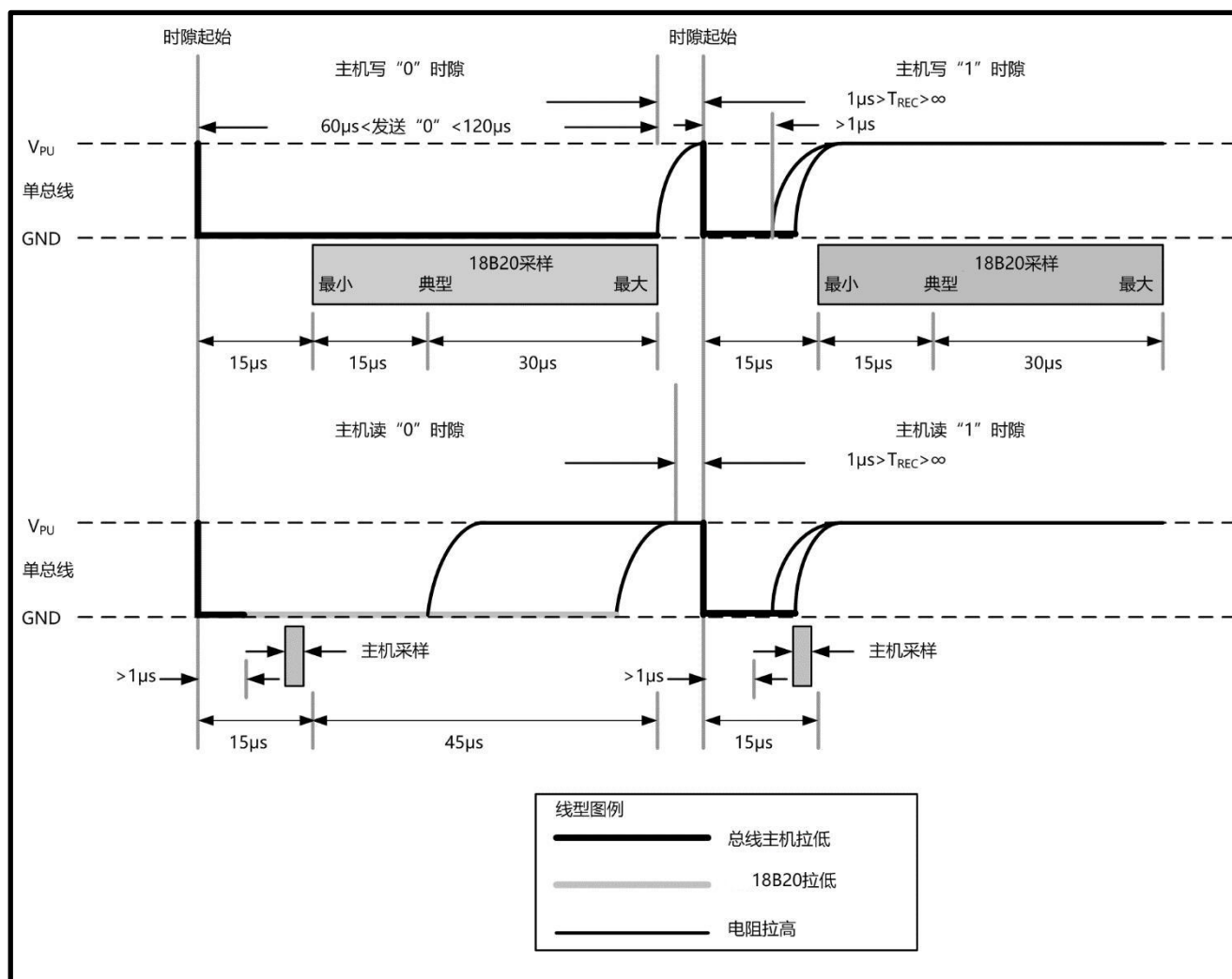
图 14 读/写时序
