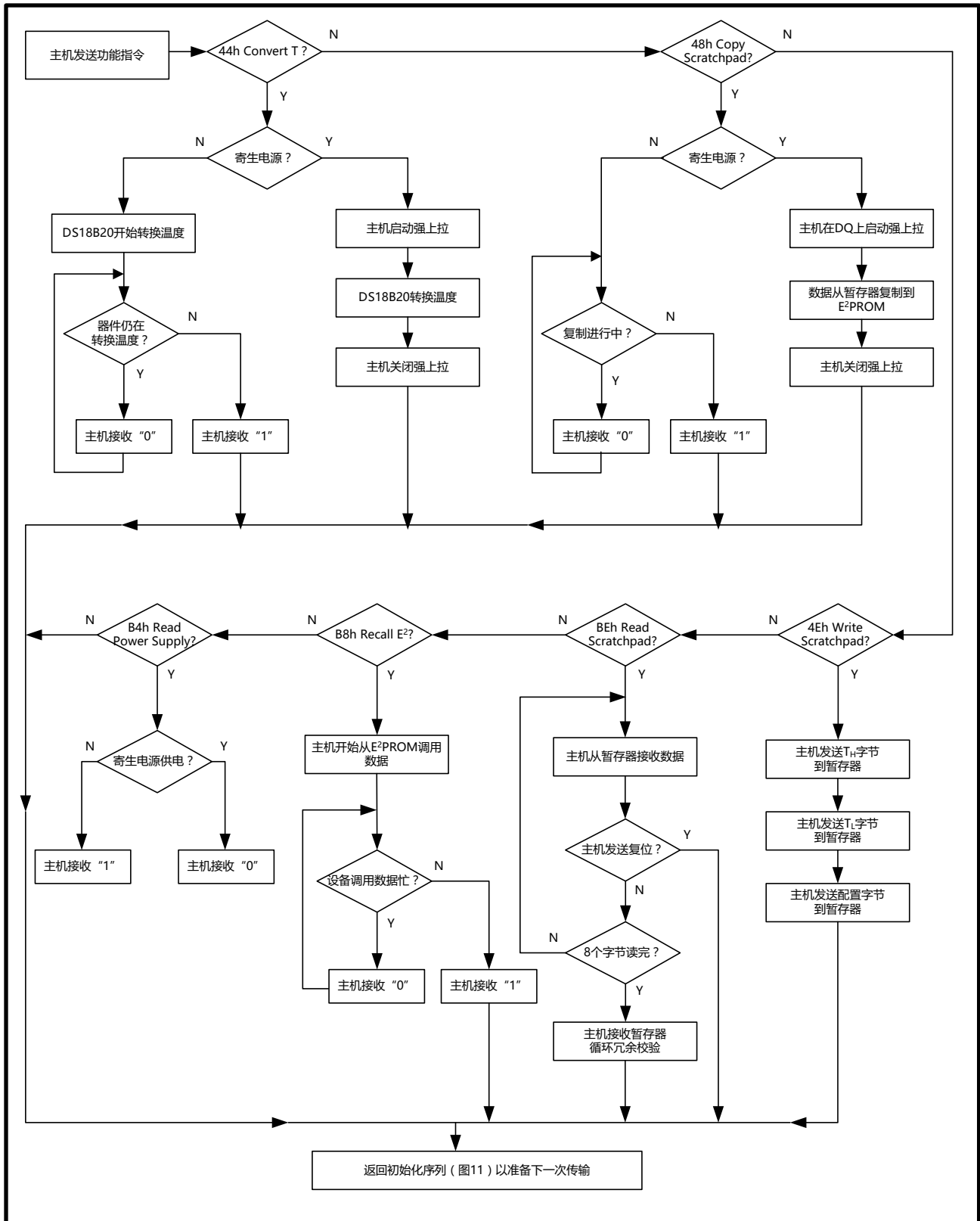
图 12 DS18B20 功能指令流程图
