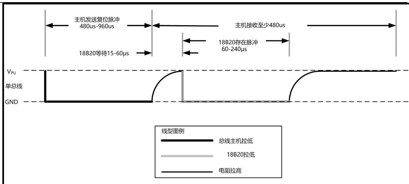
图 13 初始化时序
