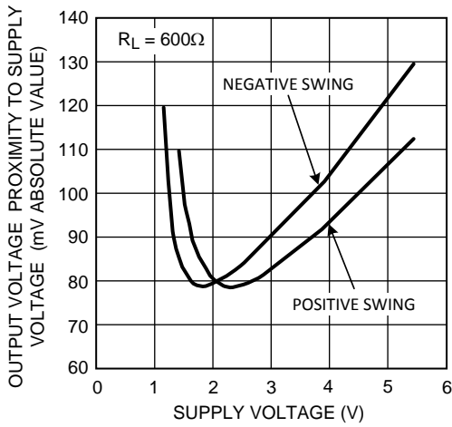
图 7. 输出电压摆幅与电源电压间的关系
