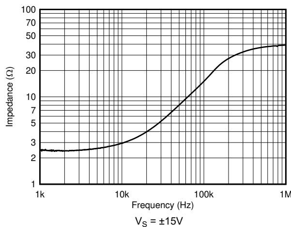
V_S = \pm 15\text{V} 开环输出阻抗
