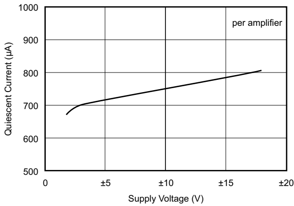
静态电流与电源电压间的关系
