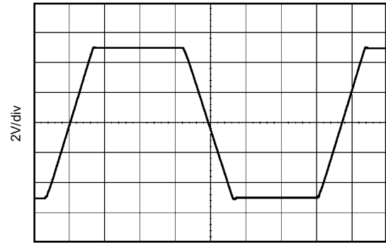
10µs/div G = 1, C_L = 1500\text{pF} , V_S = \pm 15\text{V} 大信号阶跃响应
