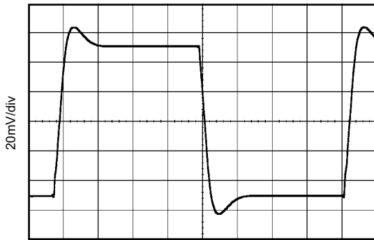
1µs/div G = 1, C_L = 0 , V_S = \pm 15\text{V} 小信号阶跃响应
