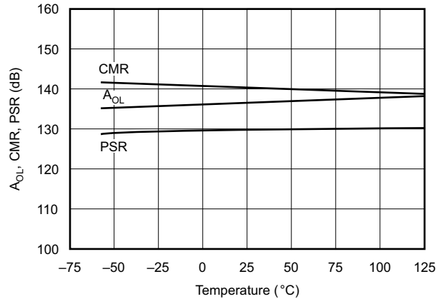
A_{OL} 、CMR、PSR 与温度间的关系
