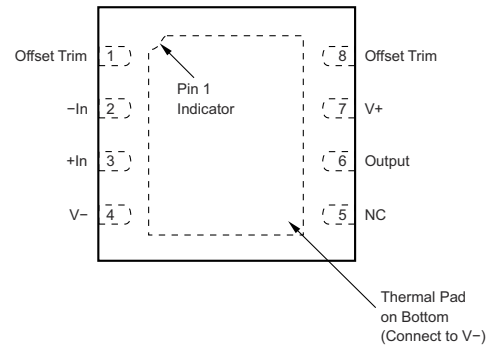
OPA277 SOP-8封装 (顶视图)
