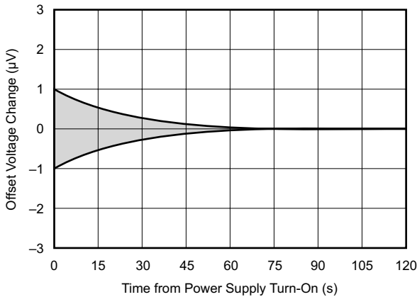
预热失调电压温漂
