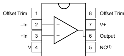
OPA277 P 封装，SOP-8封装
