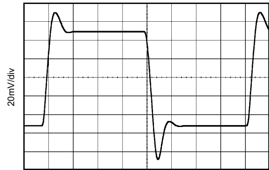
1µs/div G = 1, C_L = 1500\text{pF} , V_S = \pm 15\text{V} 小信号阶跃响应
