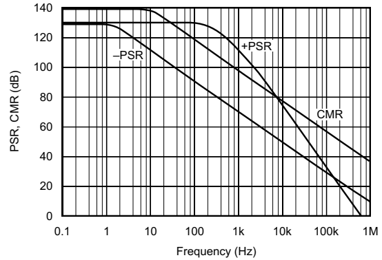
电源和共模抑制与频率间的关系
