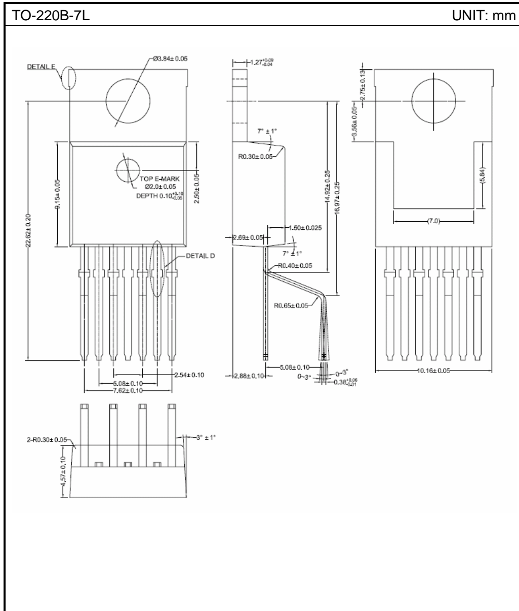
封装外形图
