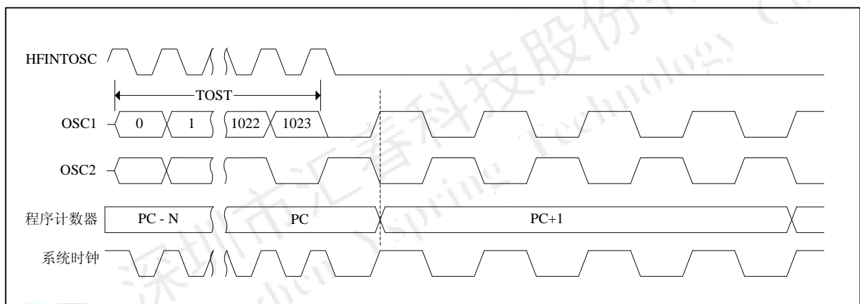
图 4-7-3: 双速启动
