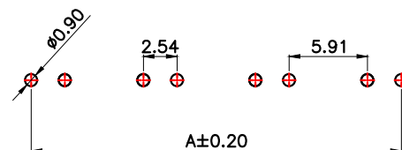
适用线路板 (PCB LAYOUT)
