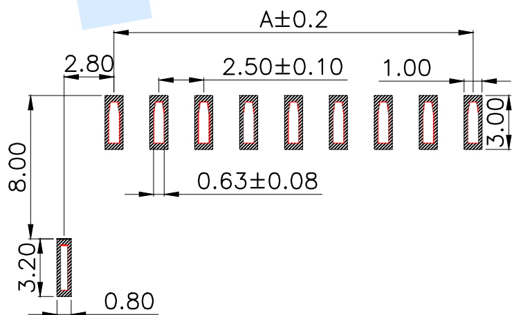
适用线路板(PCB LAYOUT)
