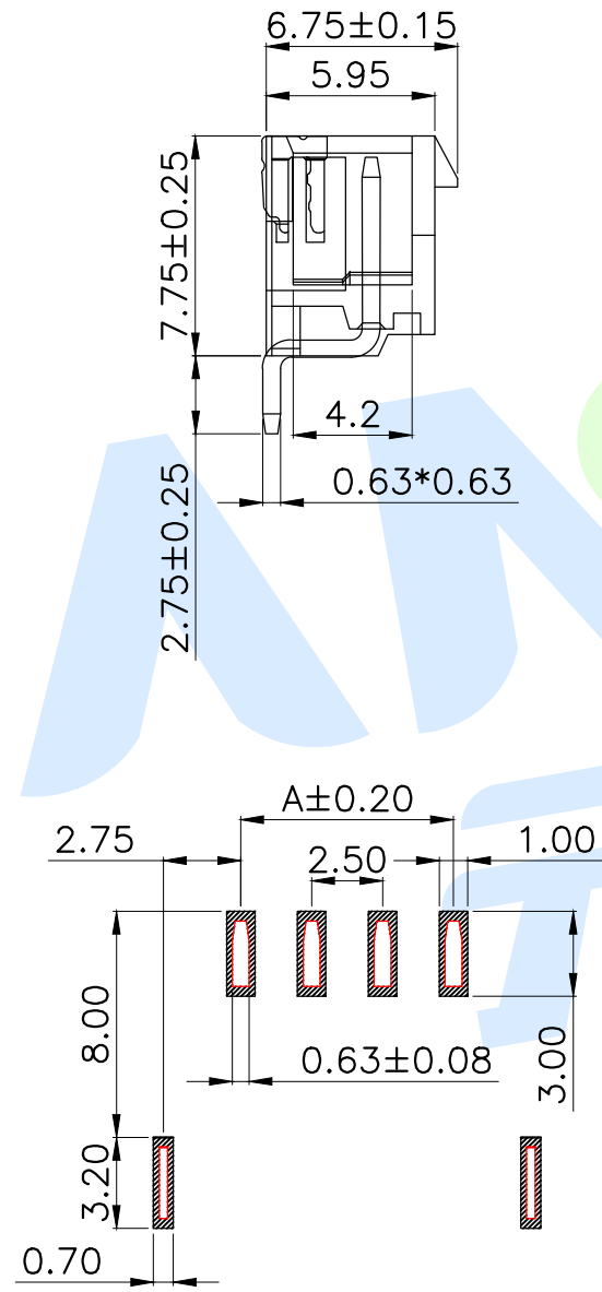
适用线路板 (PCB LAYOUT)
