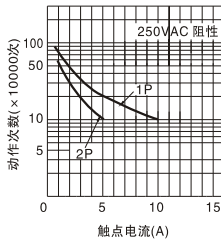
寿命曲线
