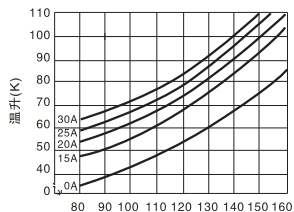
线圈电压额定值的百分比
