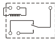
接线图(底视图)
