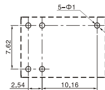
安装孔位图(底视图)
