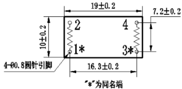
底视图
