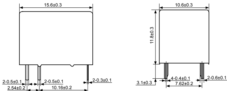
外形图
