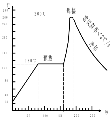
图 5 再流焊焊接曲线
