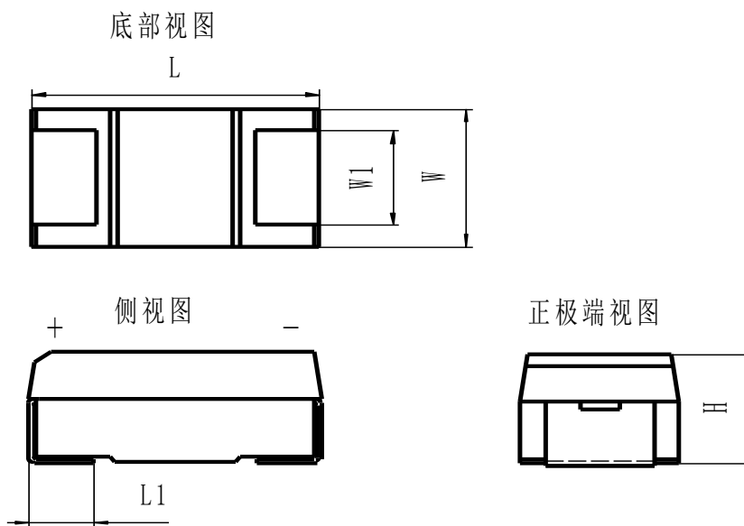
图 1 外形图
