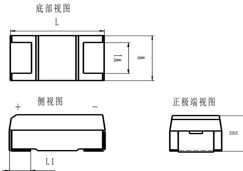
图 1 外形图
