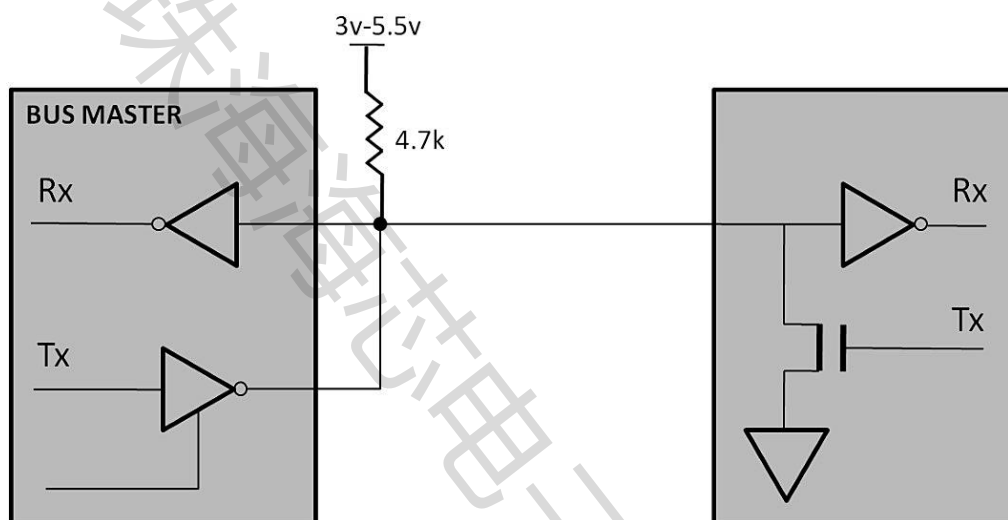
图 20 HX18B20-T 与主机连接示意图
