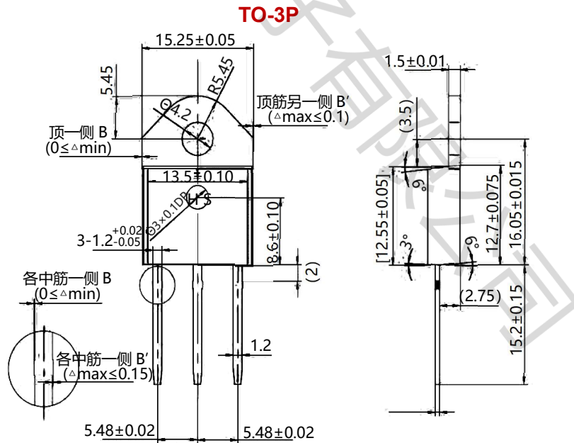
外形尺寸图
