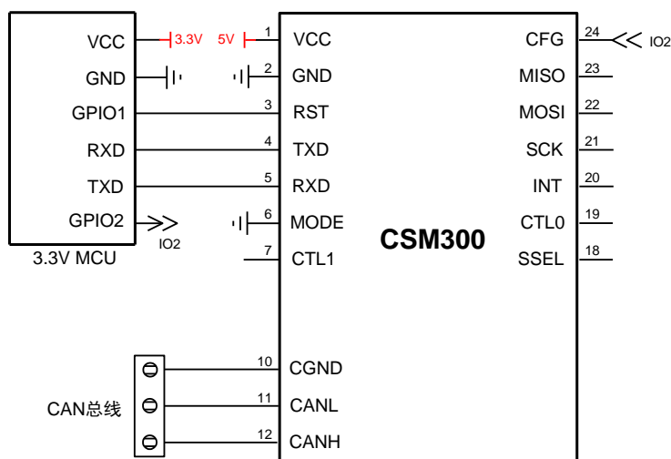
图 2.6 UART 转 CAN 参考电路 (CSM300)
