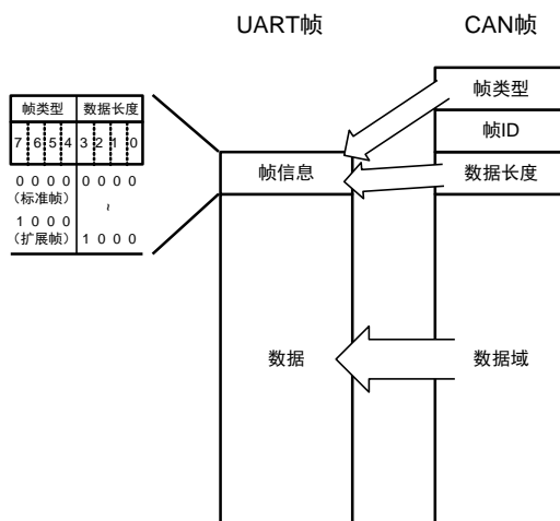
图 3.14 CAN 帧转 UART 帧（透明转换，帧信息使能）
