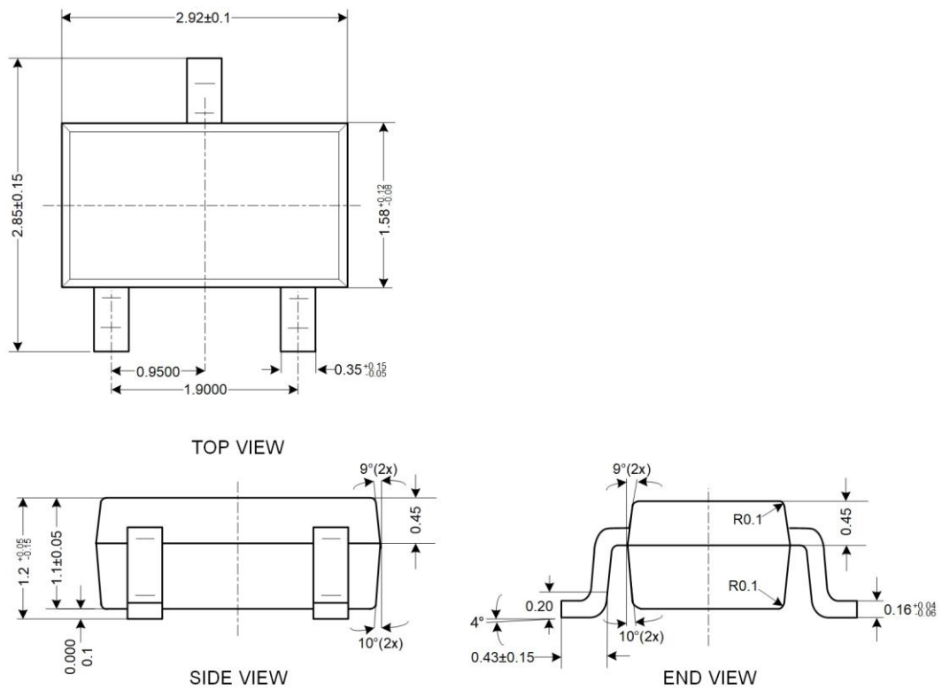
图 5.1 封装尺寸图
