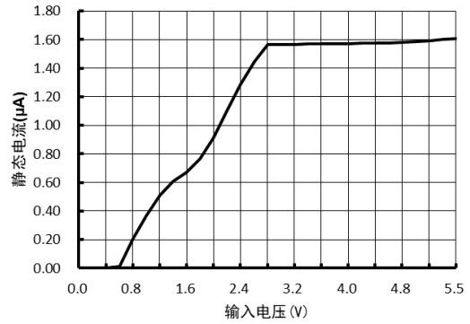
图 2.3 静态电流与输入电压关系 ( I_{OUT}=0mA )
