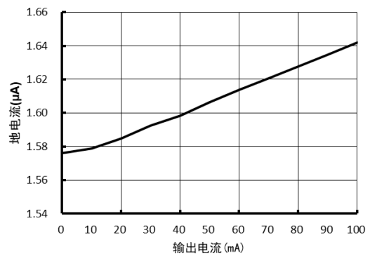
图 2.7 地电流与负载电流的关系
