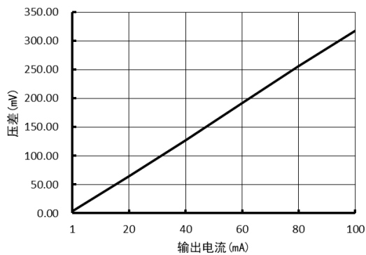
图 2.6 压差与负载电流的关系
