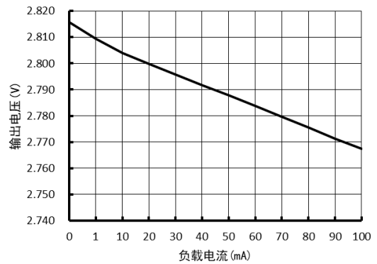
图 2.5 负载调整特性 ( V_{IN}=4.8V )
