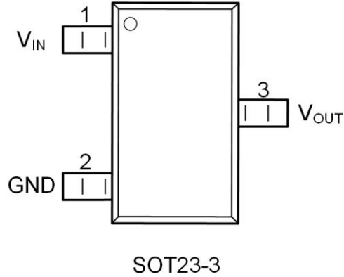
图 2.1 管脚信息
