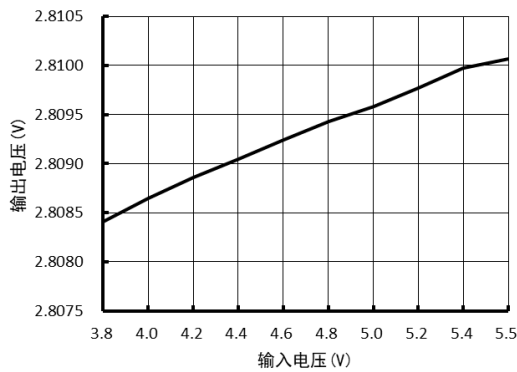
图 2.4 线性调整特性
