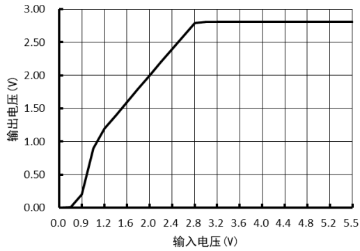
图 2.2 输入输出电压特性
