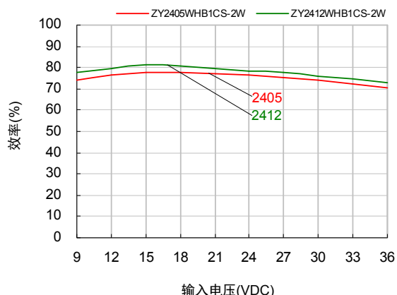
效率与输入电压关系曲线图
