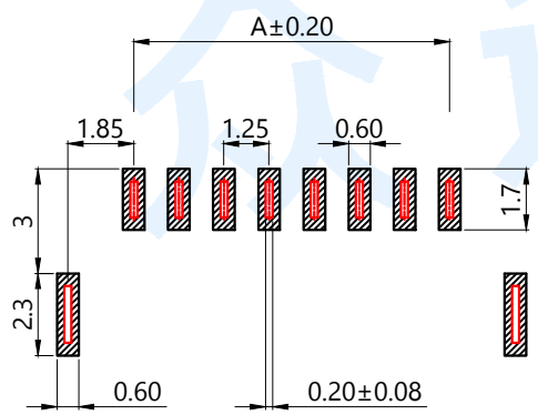
适用线路板 (PCB LAYOUT)
