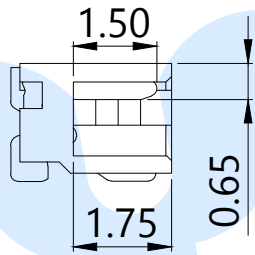
剖面E-E
