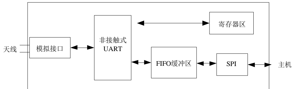
图 1. Ci522 简化框图
