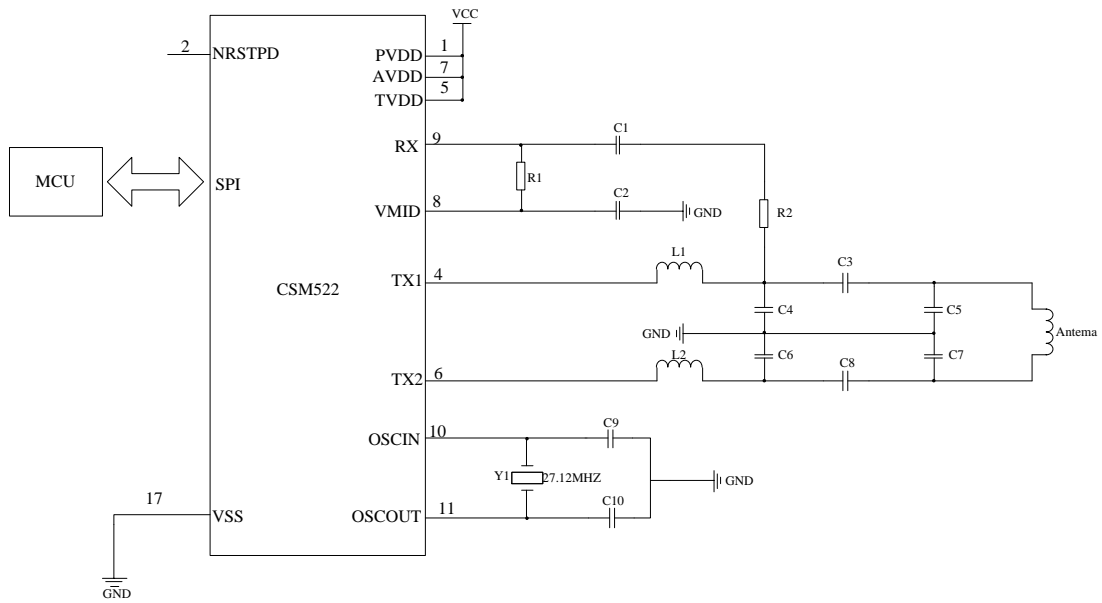
图 10. 典型应用图-2
