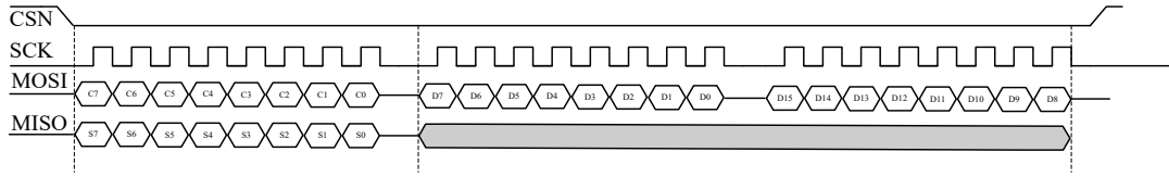
图 7.4 SPI 写
