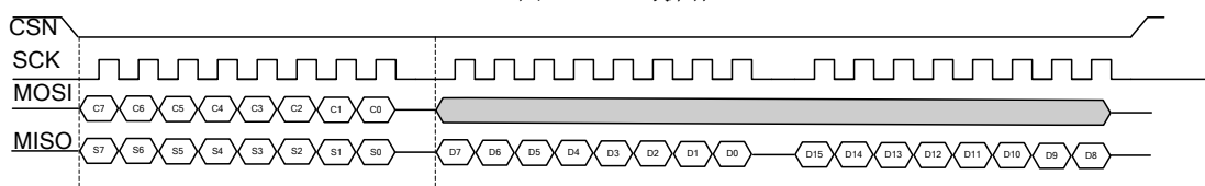
图 5-2 SPI 读操作
